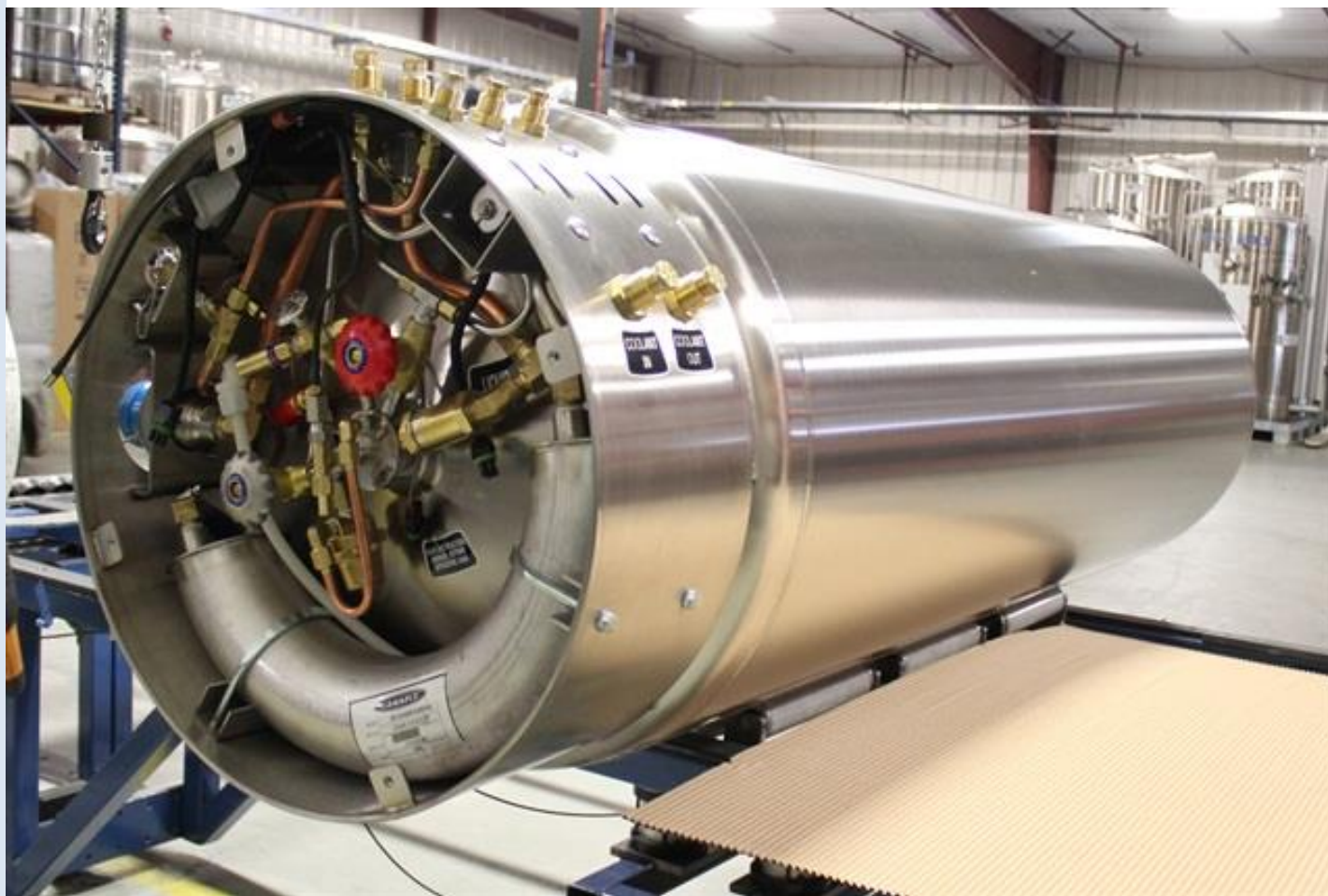
Sistema de propulsión para gas natural licuado
