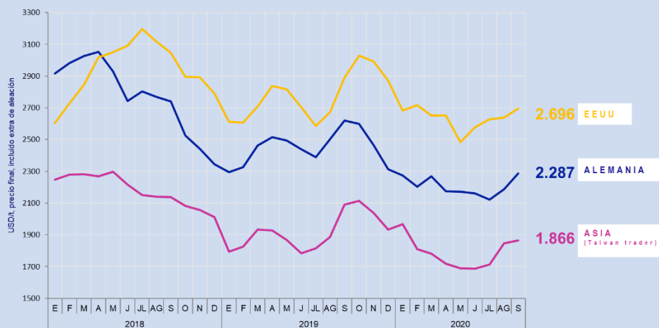
Precios de la chapa de acero inoxidable, AISI 304 laminada en frío 2,0mm (fuente: CRU)
